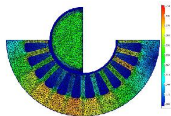
高速永磁电机电磁有限元分析
