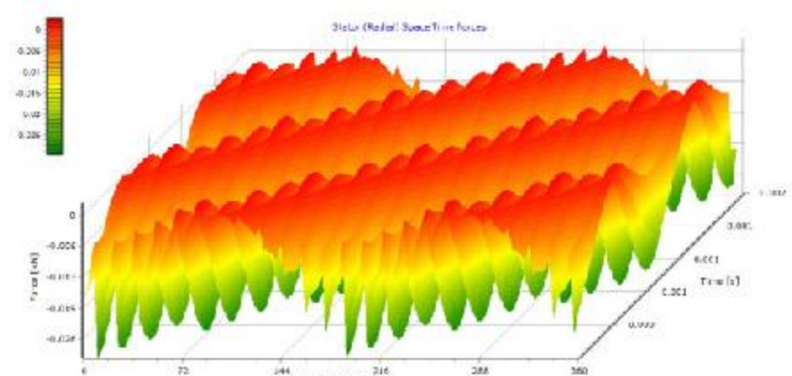
高速永磁电机2D时域扭矩分布
